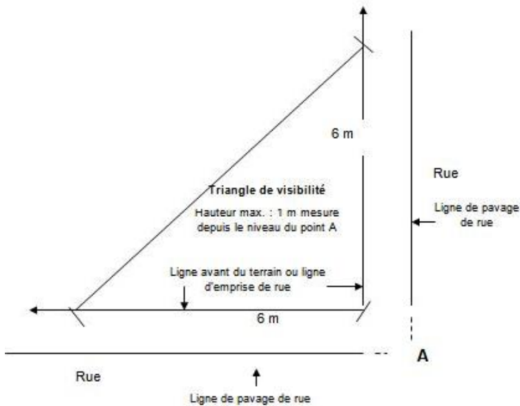
Figure 6 - Triangle de visibilité
