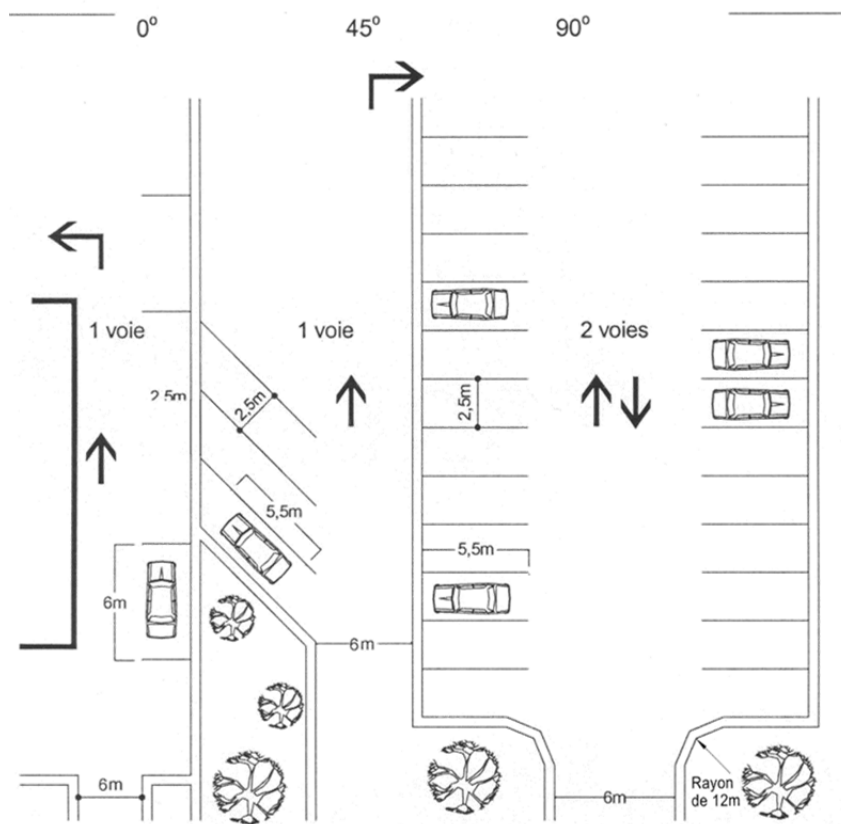
Figure 11 - Dimension d'une case de stationnement avec angle
