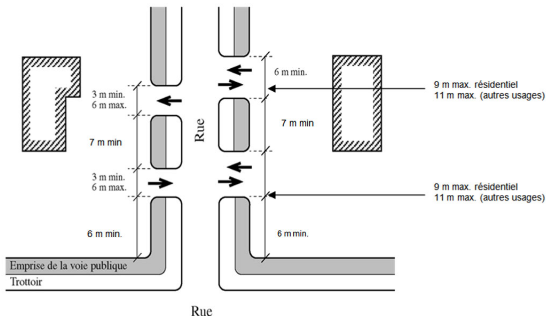
Figure 12 - Accès véhiculaire
