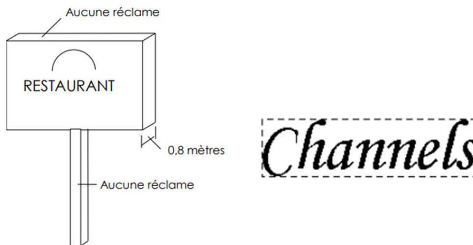
Figure 14 – Calcul de l’aire d’une enseigne
