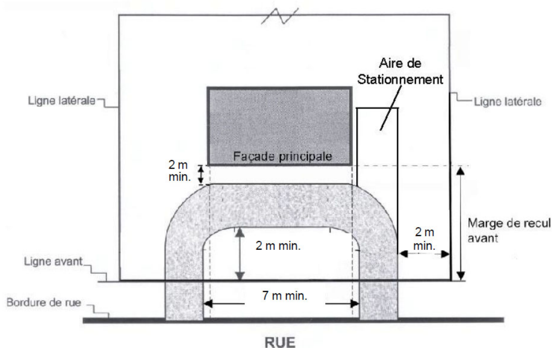
Figure 13 - Accès en demi-cercle
